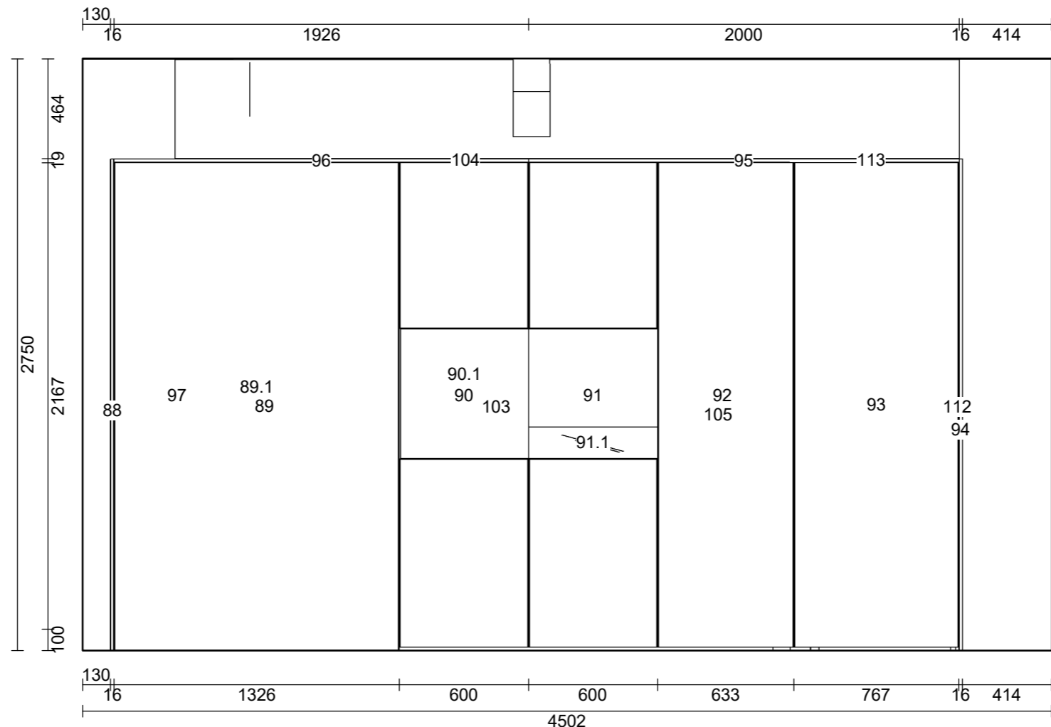
Elevation G
