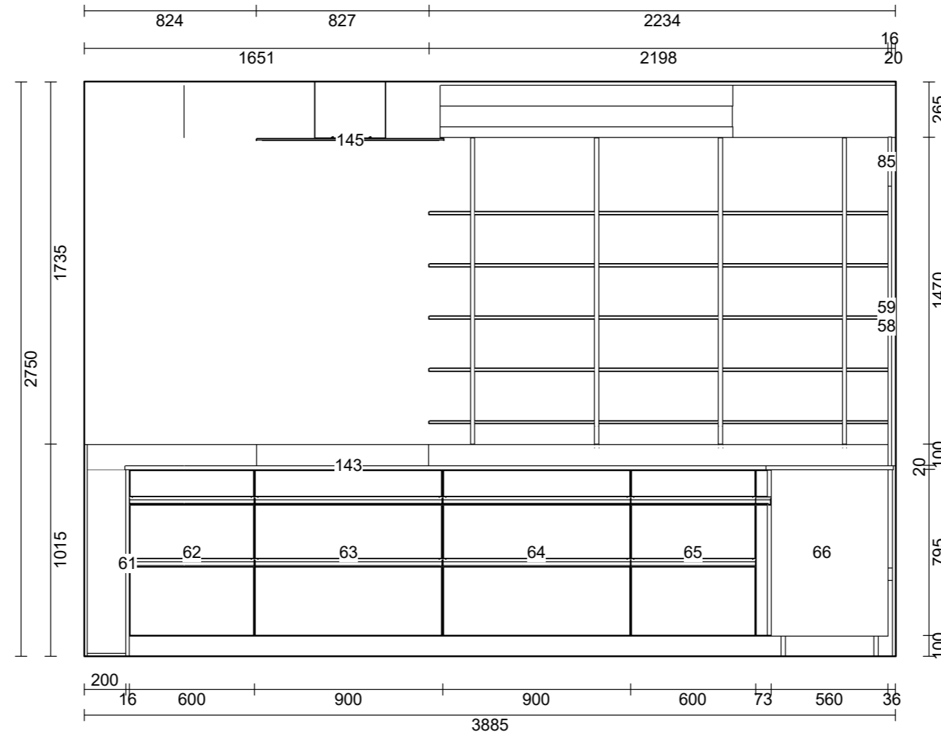
Elevation E
