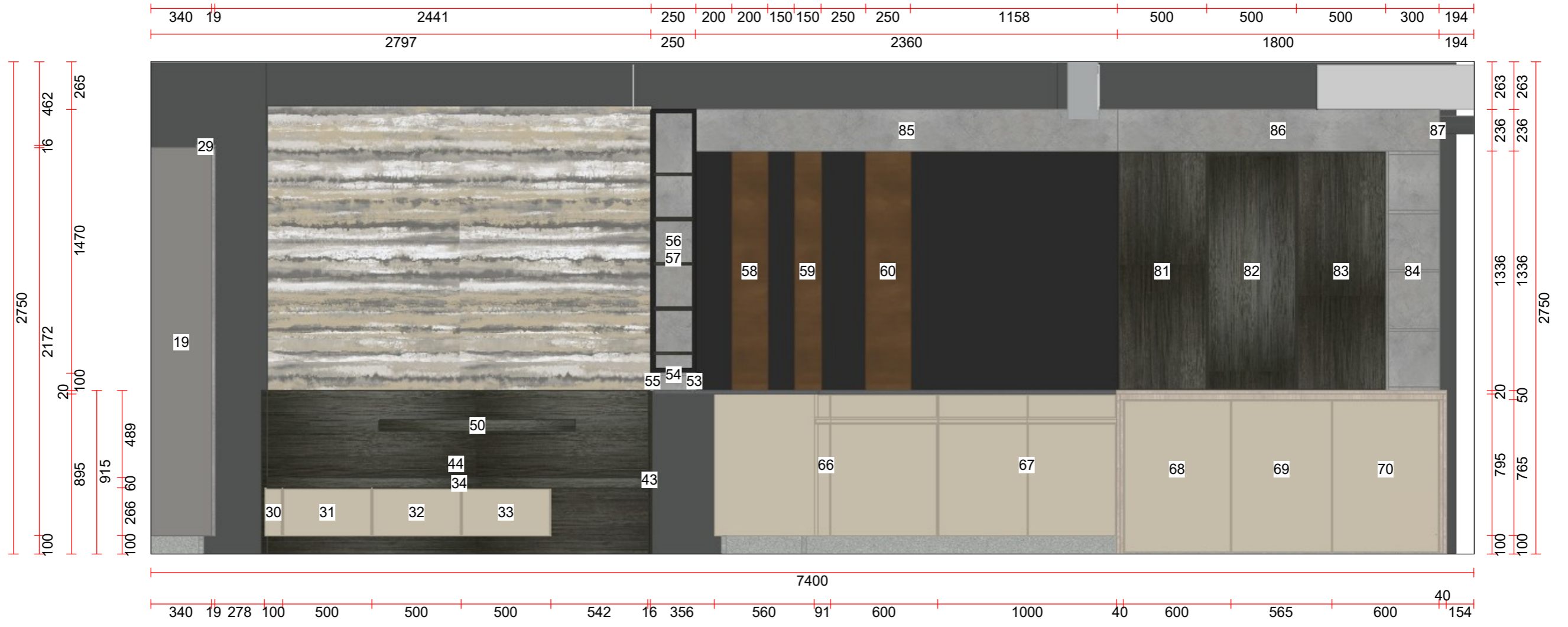
Elevation B
