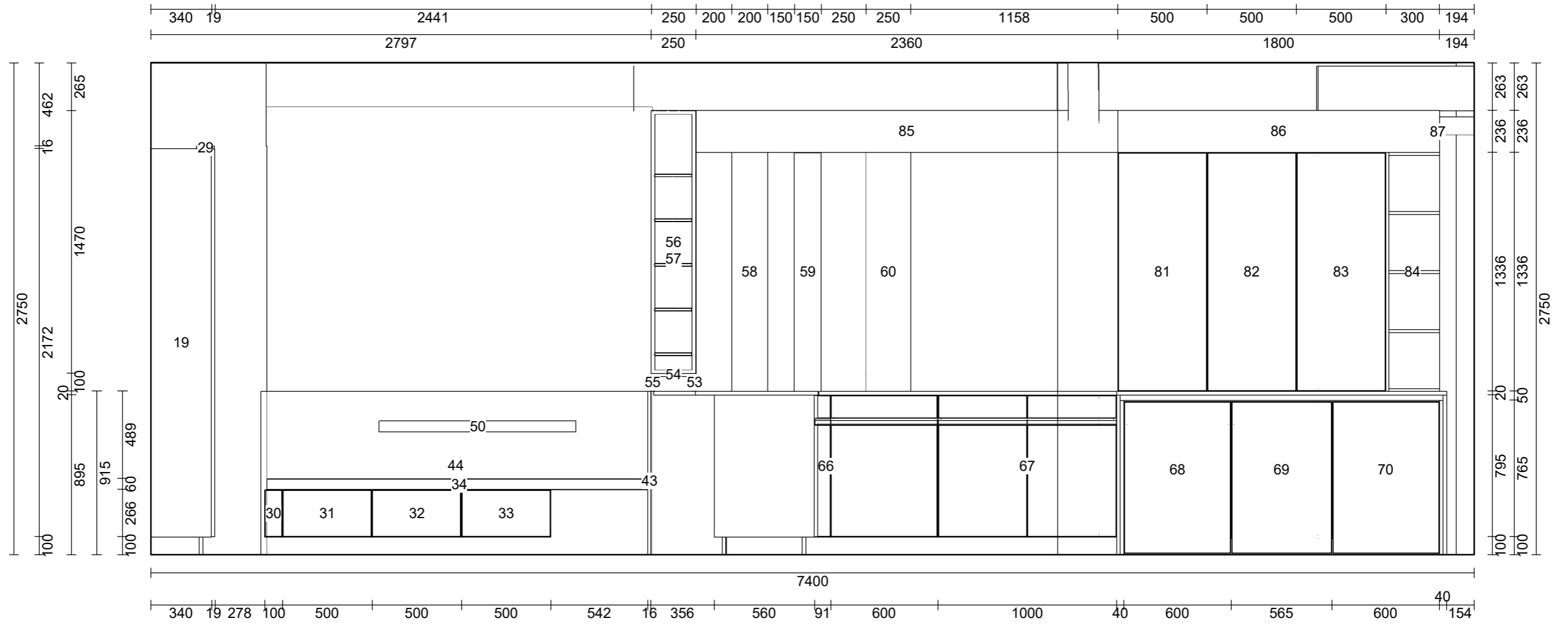
Elevation B
